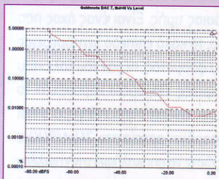
Αρμονική παραμόρφωση και θόρυβος σε συνάρτηση με την στάθμη. Σήμα: 997Hz
