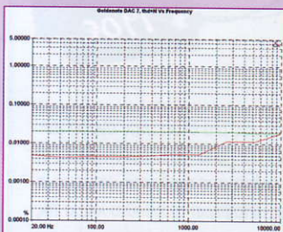
Αρμονική παραμόρφωση και θόρυβος σε συνάρτηση με την συχνότητα. Στάθμες: -1dBFS (κόκκινη καμπύλη) και -20dBFS (πράσινη καμπύλη)
